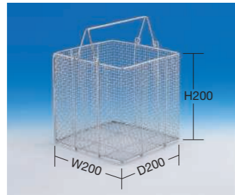
ステンレスSUS304 線径網：0.8mm 線径枠：3mm（単位：mm） 外形寸法(W×D×H) □品番 価格(税抜) メーカー希望小売価格 200×200×200 194615 SS角カゴ200 ¥4,370 ¥5,900 ●網目5.5mm目 ●規定出荷数：18個
