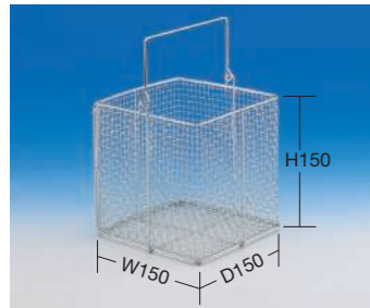
ステンレスSUS304 線径網：0.8mm 線径枠：3mm（単位：mm） 外形寸法(W×D×H) □品番 価格(税抜) メーカー希望小売価格 150×150×150 194614 SS角カゴ150 ¥3,130 ¥4,600 ●網目5.5mm目 ●規定出荷数：24個
