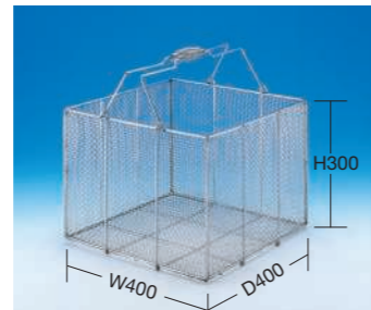
ステンレスSUS304 線径網：0.95mm 線径枠：4mm（単位：mm） 外形寸法(W×D×H) □品番 価格(税抜) メーカー希望小売価格 400×400×300 194609 SS角カゴ443 ¥15,520 ¥22,500 ●網目5.5mm目 ●規定出荷数：4個
