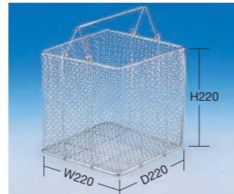
ステンレスSUS304 線径網：0.8mm 線径枠：3mm（単位：mm） 外形寸法(W×D×H) □品番 価格(税抜) メーカー希望小売価格 220×220×220 194618 SS角カゴ220 ¥5,320 ¥7,700 ●網目5.5mm目 ●規定出荷数：12個
