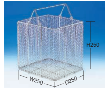
ステンレスSUS304 線径網：0.8mm 線径枠：4mm（単位：mm） 外形寸法(W×D×H) □品番 価格(税抜) メーカー希望小売価格 250×250×250 194606 SS角カゴ250 ¥7,090 ¥9,300 ●網目5.5mm目 ●規定出荷数：4個
