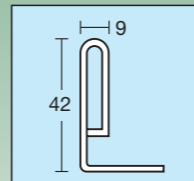
●棚板断面図
