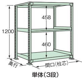
単体(3段)
