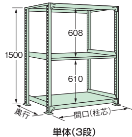
単体(3段)
