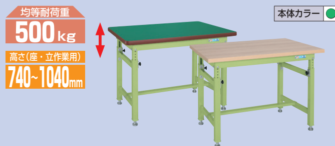
ギヤー式昇降作業台 固定式
